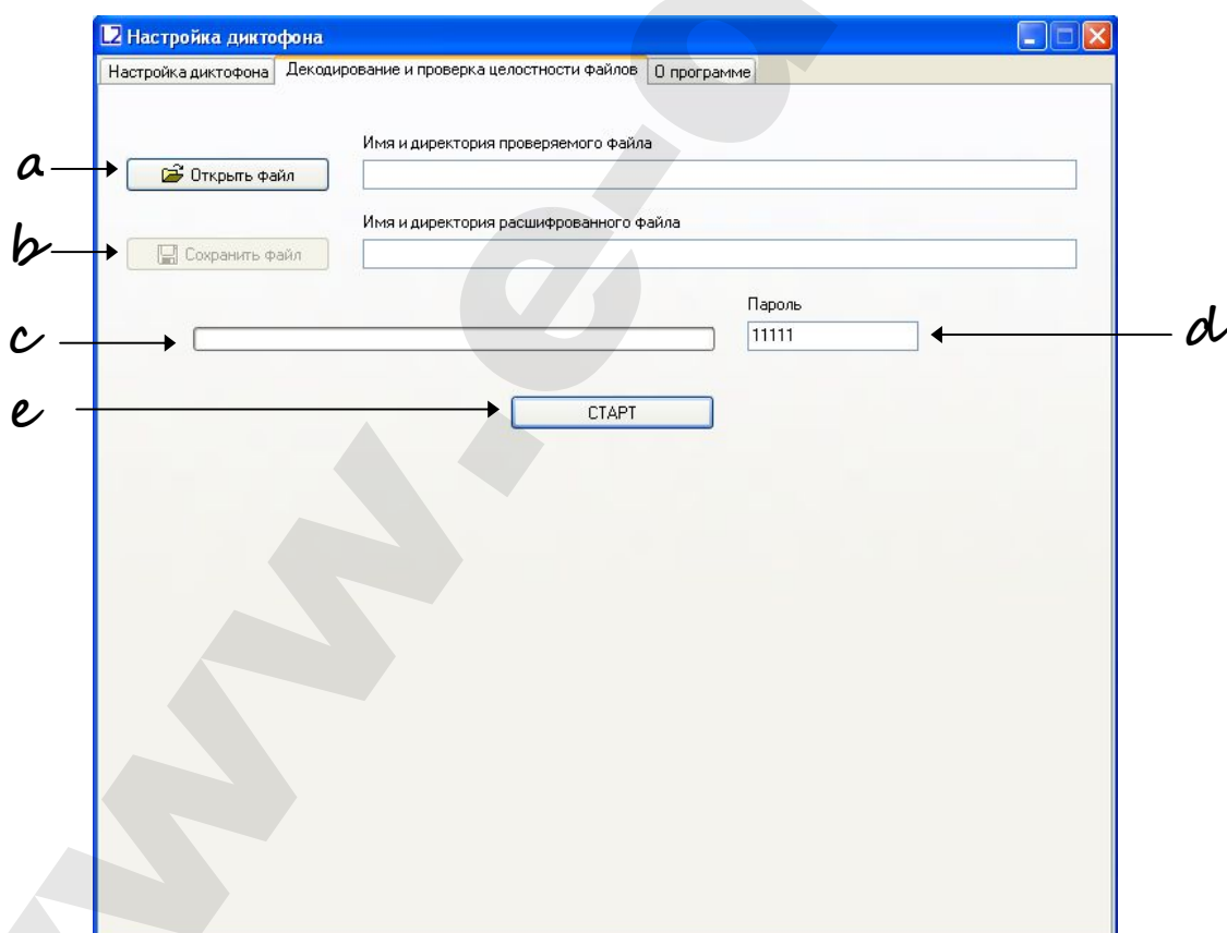
Рис. 4. Окно проверки цифровой подписи файлов и их декодирования.
