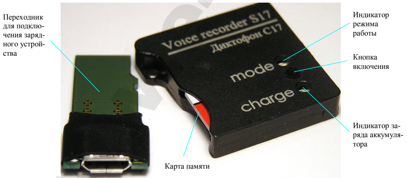
Рис. 2. Внешний вид диктофона «СОРОКА-17».
